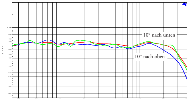
Frequenzgang: Fast keine Interferenzen, horizontal ± 10°
