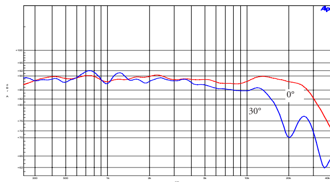
Frequenzgang: Auch 30° aus der Achse vertikal, sehr linear, exzellente Abstrahlung dank APC. MK 3- System.
