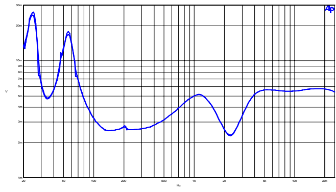
Lautsprecher: Impedanzkurve
